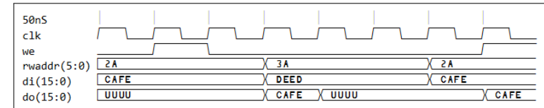
Διάγραμμα χρονισμού
