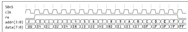
Διάγραμμα χρονισμού
