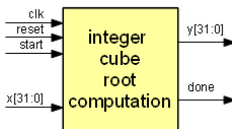
Σχήμα 2: Η διεπαφή του κυκλώματος υπολογισμού ακέραιας προσέγγισης κυβικής ρίζας.
