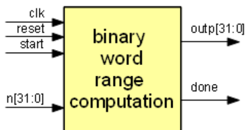
Σχήμα 2: Η διεπαφή του κυκλώματος υπολογισμού του εύρους δυαδικής λέξης.
