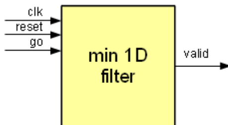
Σχήμα 2: Η διεπαφή του κυκλώματος φίλτρου ελαχίστου.
